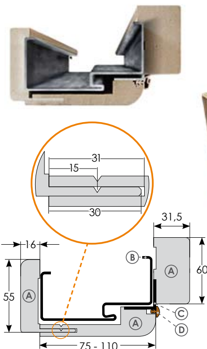
ROZMĚRY VE SVĚTLOSTI KOVOVÉ ZÁRUBNĚ / ROZMERY VO SVETLOSTI KOVOVEJ ZÁRUBNE (mm)
