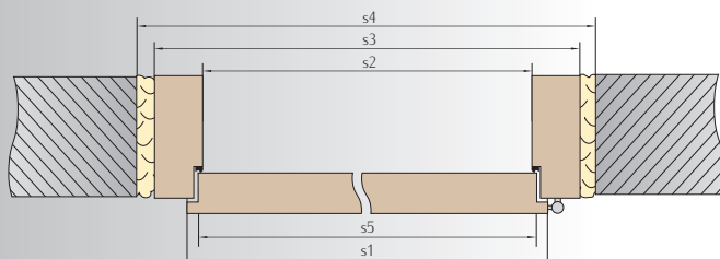
Schéma pevnej zárubne
