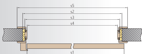
SYSTÉM MONTOVANÝ PRI POUŽITÍ REGULOVATEĽNÉHO TUNELA
