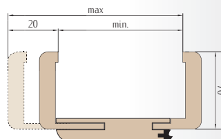
Rozsah regulácie regulovanej zárubne
